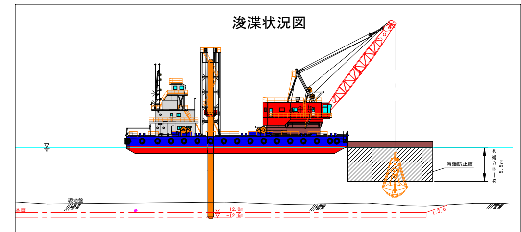
揚土状況図
