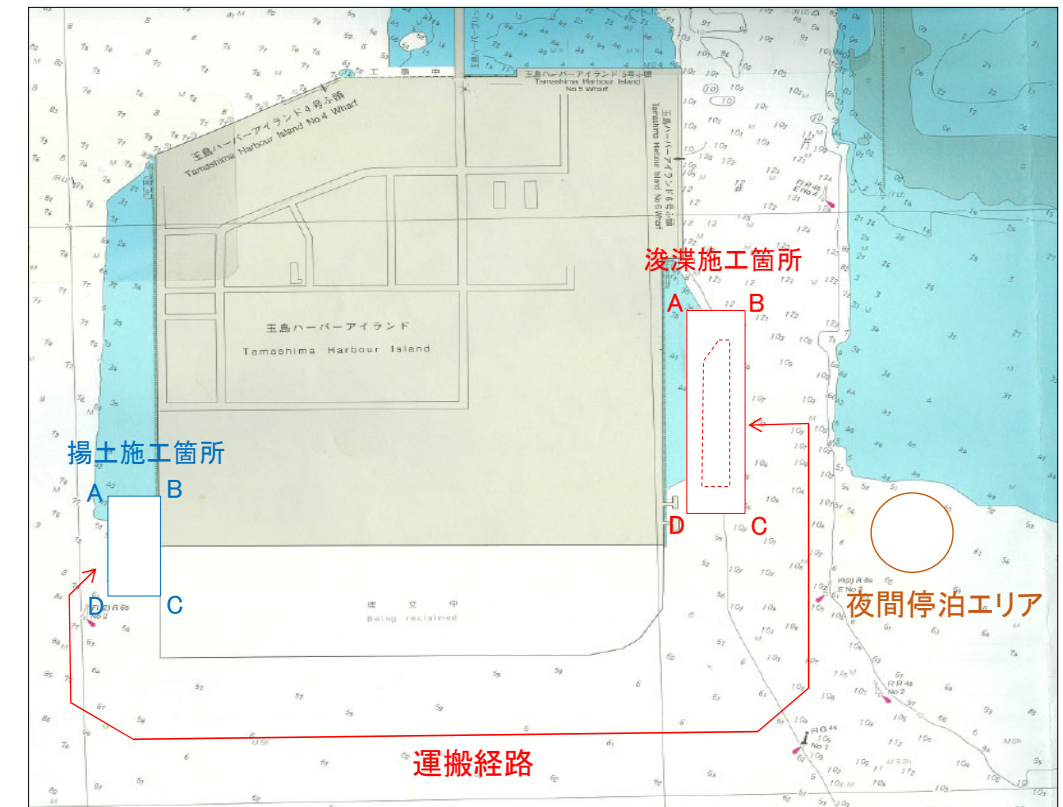
作業区域平面図
