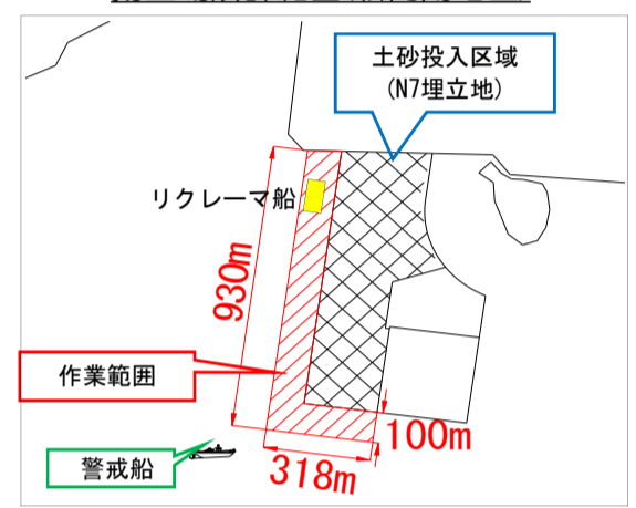
揚土場所詳細図(新南陽地区)
