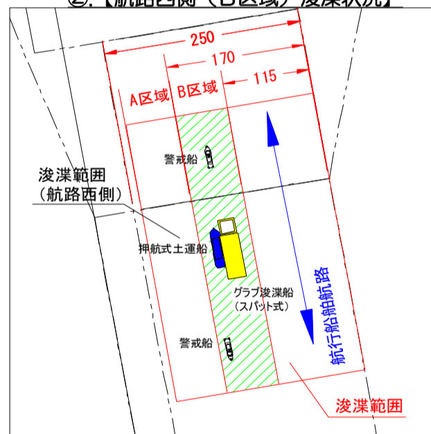
②.【航路西側（B区域）浚渫状況】
