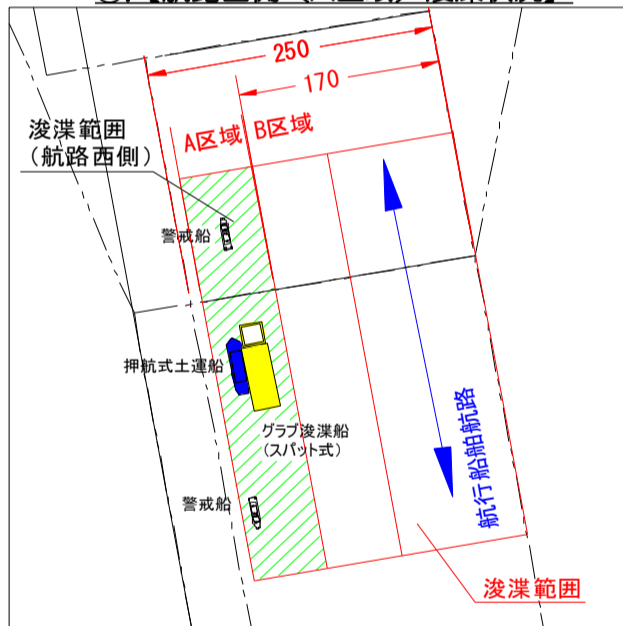
①.【航路西側（A区域）浚渫状況】
