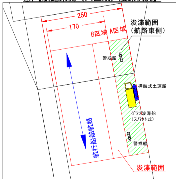
③.【航路東側（A区域）浚渫状況】
