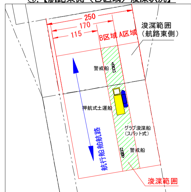
④.【航路東側（B区域）浚渫状況】
