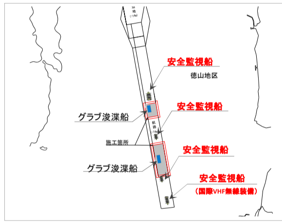
浚渫場所詳細図(徳山地区)
