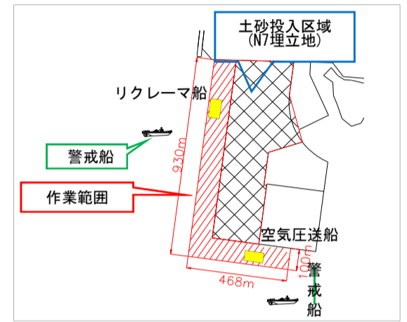
揚土場所詳細図(新南陽地区)
