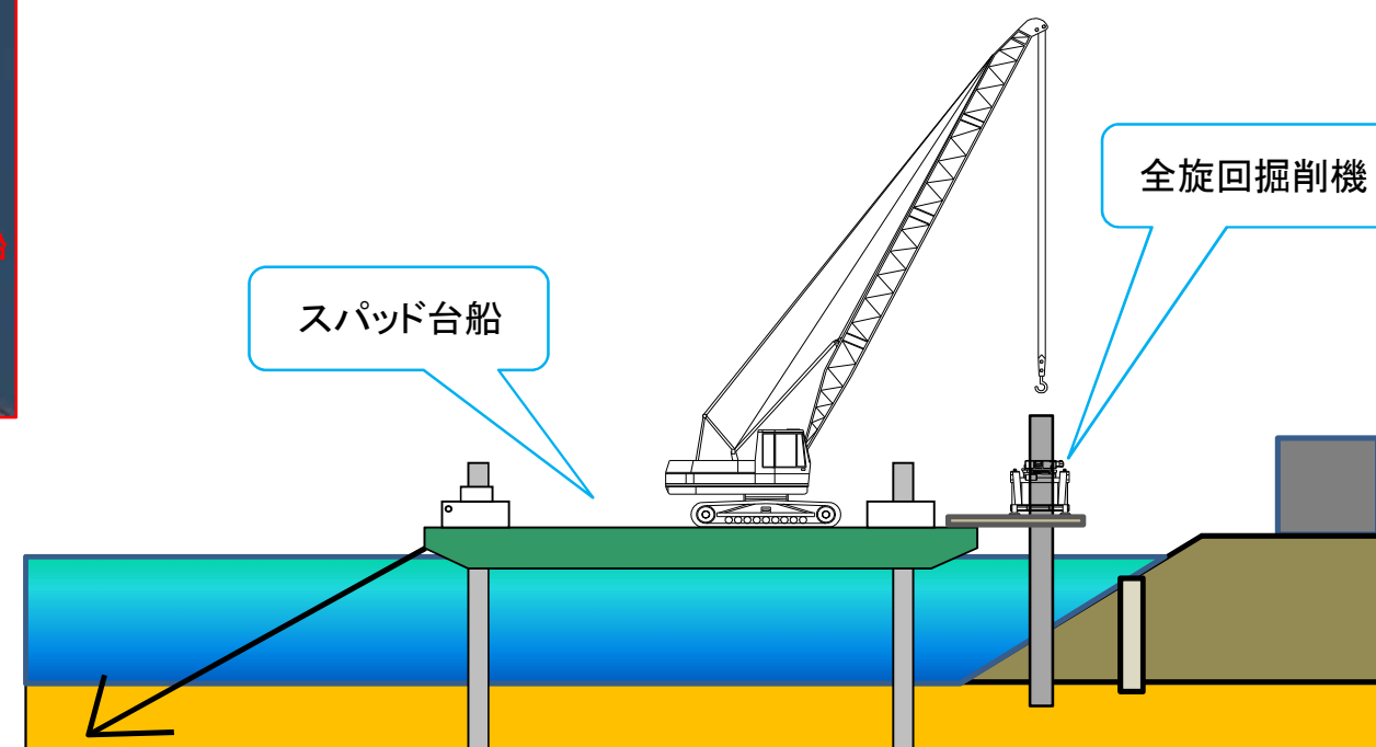
先行掘削作業状況図
