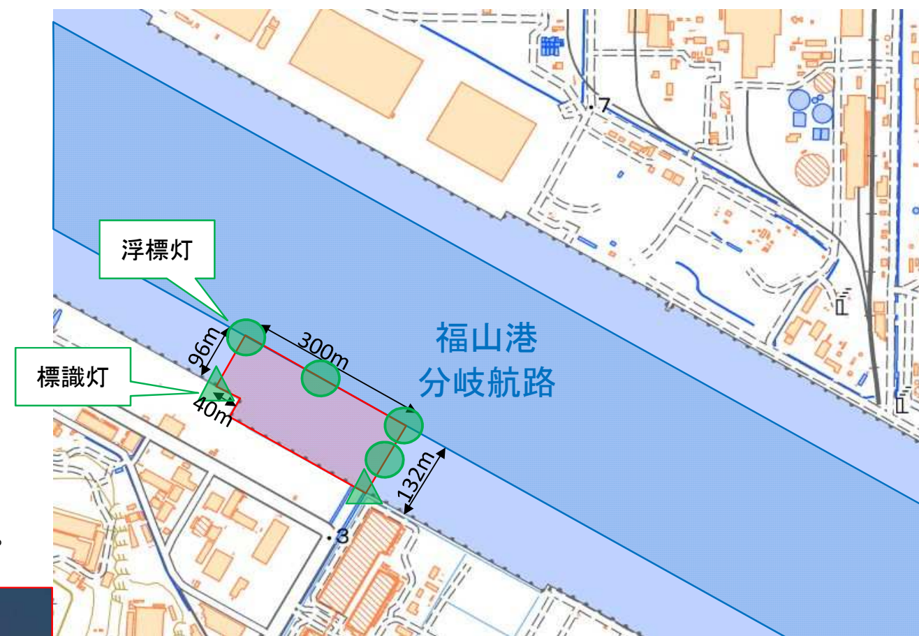
図-2 作業区域詳細図
