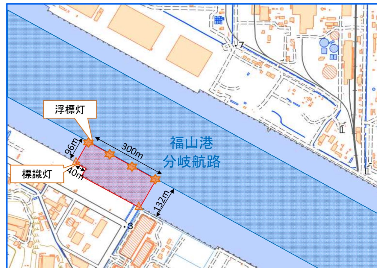
図-2 作業区域詳細図
