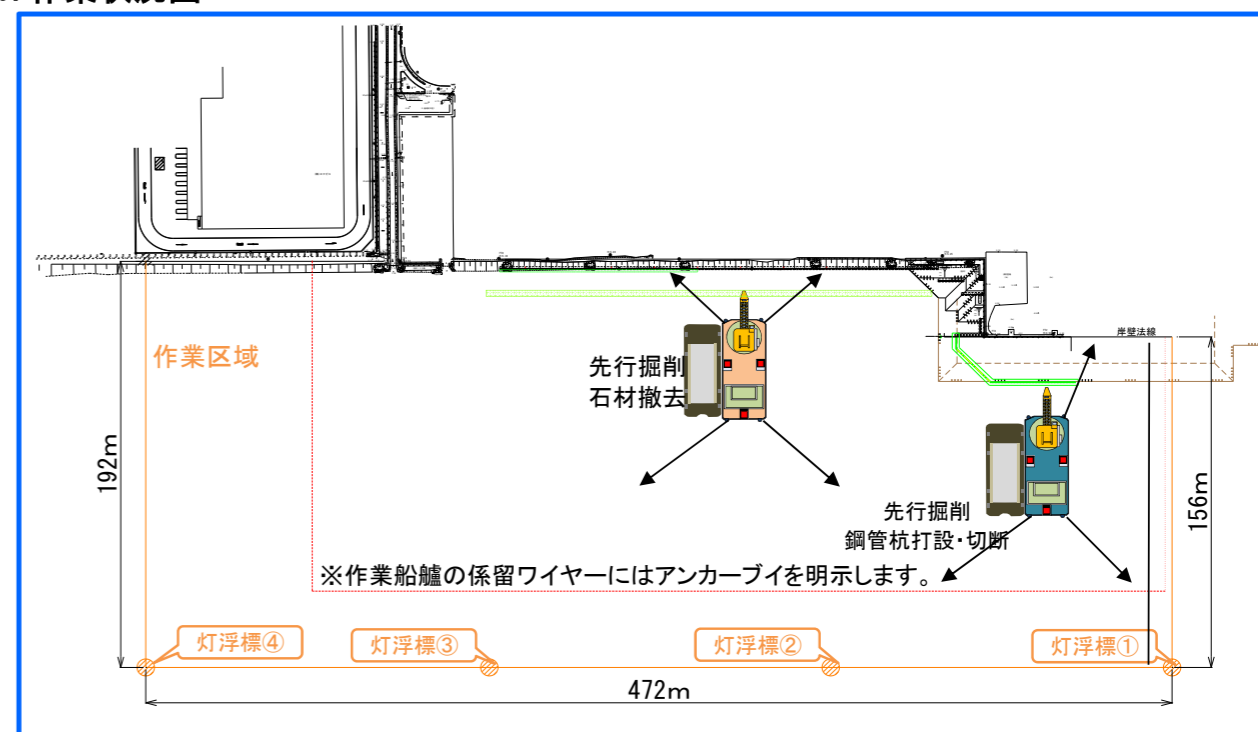
図-2 作業区域詳細図
