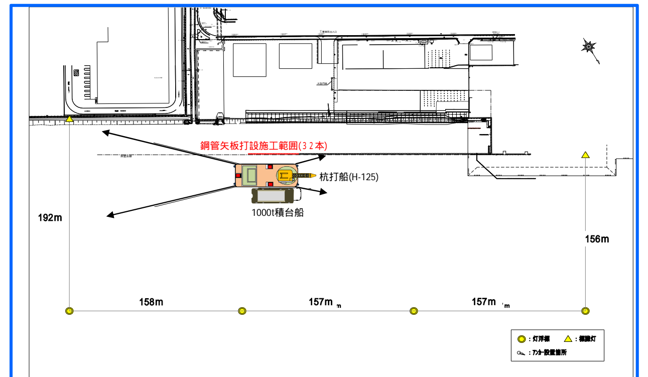
図-3 鋼管矢板打設作業状況図
