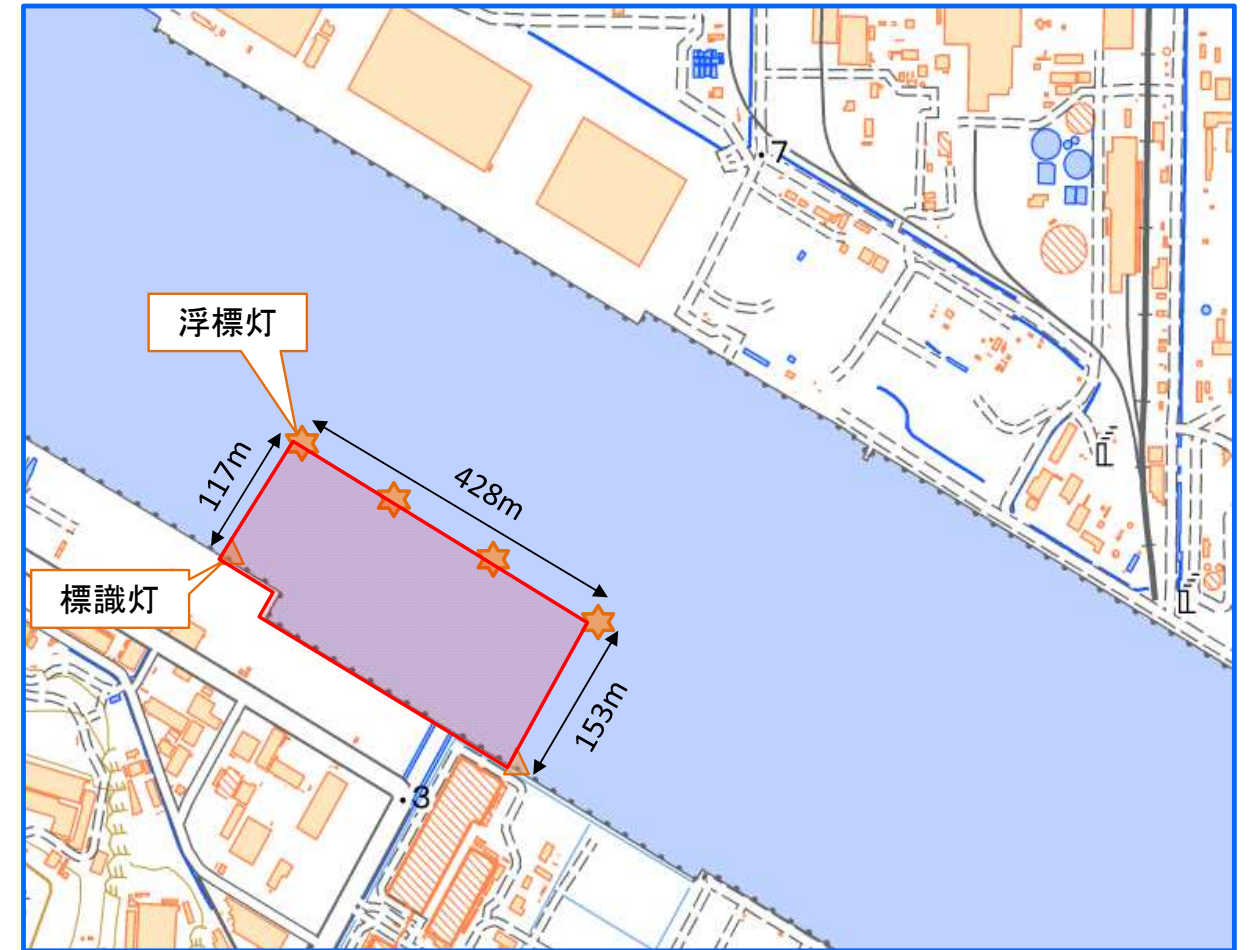
図-2 作業区域詳細図
