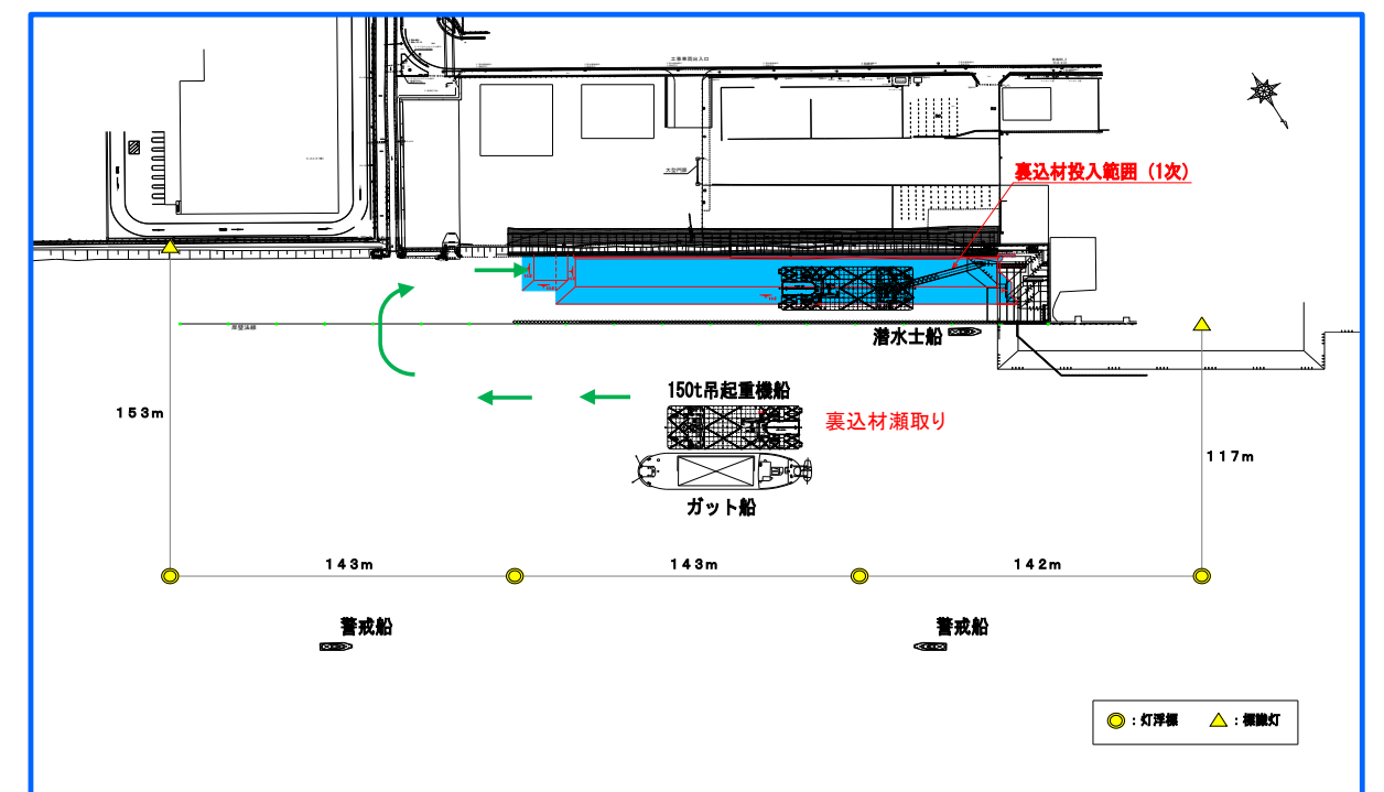
図-3 裏込材投入作業状況図
