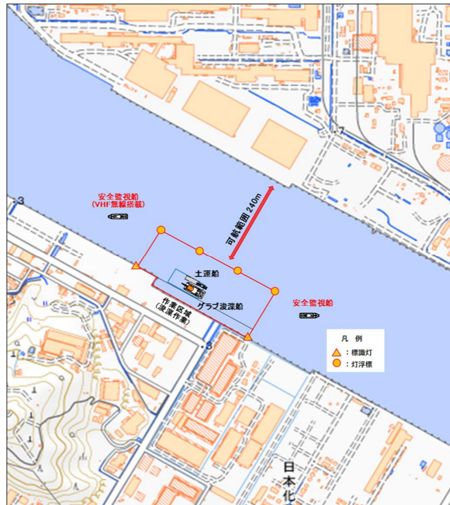
作業船配置(浚渫作業)
