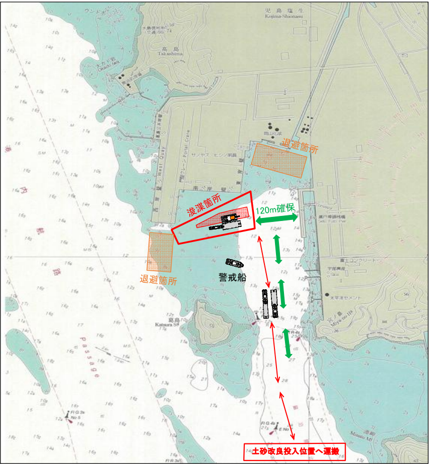
作業要領図
