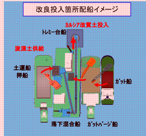
土砂改良投入作業状況図
