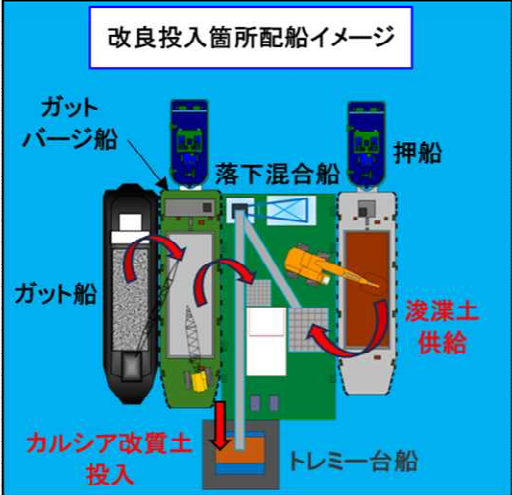
【土砂改良投入作業状況図】
